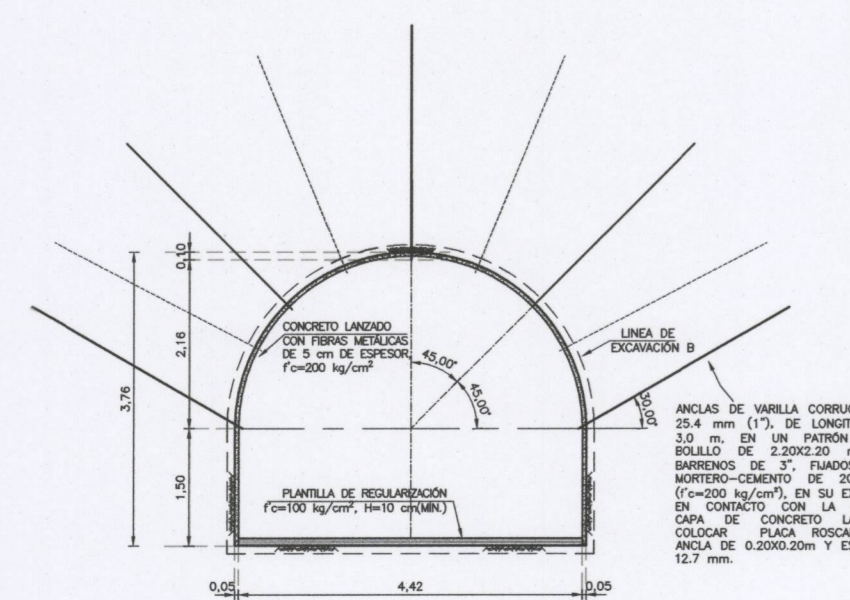
GALERÍA DE CONEXIÓN-TIPO A ESC. 1:100
