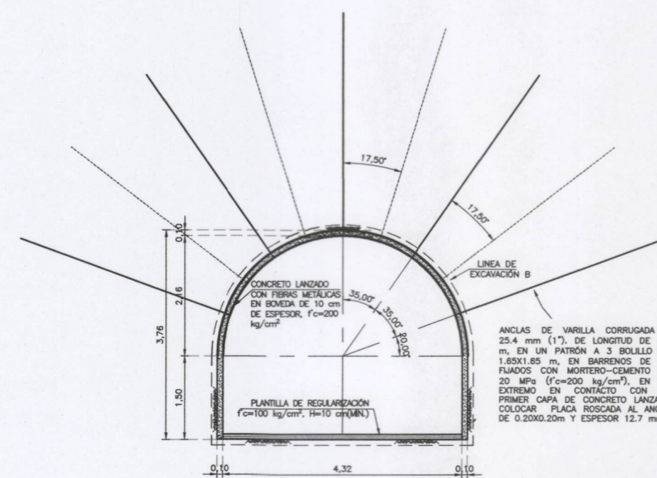
GALERÍA DE CONEXIÓN-TIPO B ESC. 1:100
