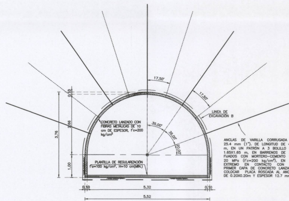
GALERÍA DE APROXIMACIÓN-TIPO B ESC. 1:100
