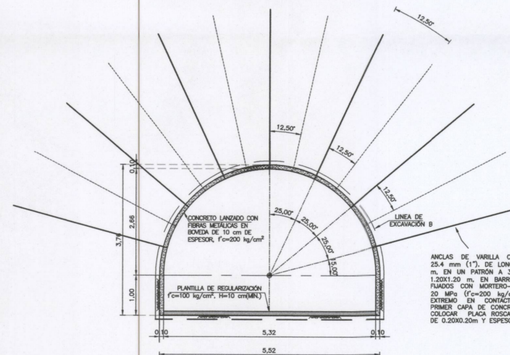
GALERÍA DE APROXIMACIÓN-TIPO C1 ESC. 1:100
