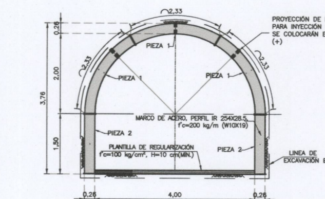
GALERÍA DE CONEXIÓN-TIPO C ESC. 1:100
