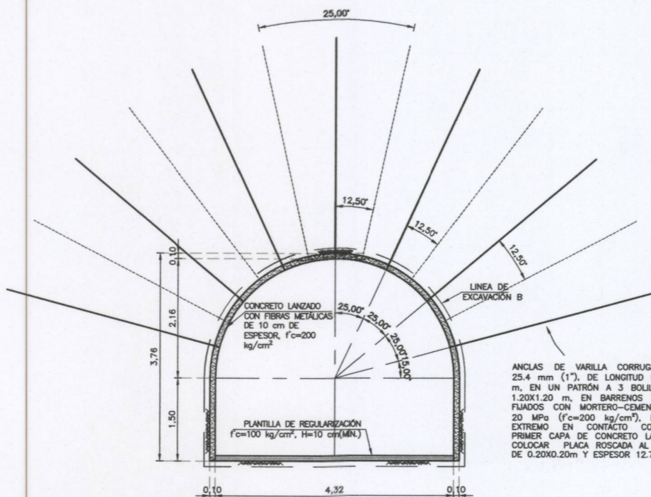
GALERÍA DE CONEXIÓN-TIPO C1 ESC. 1:100
