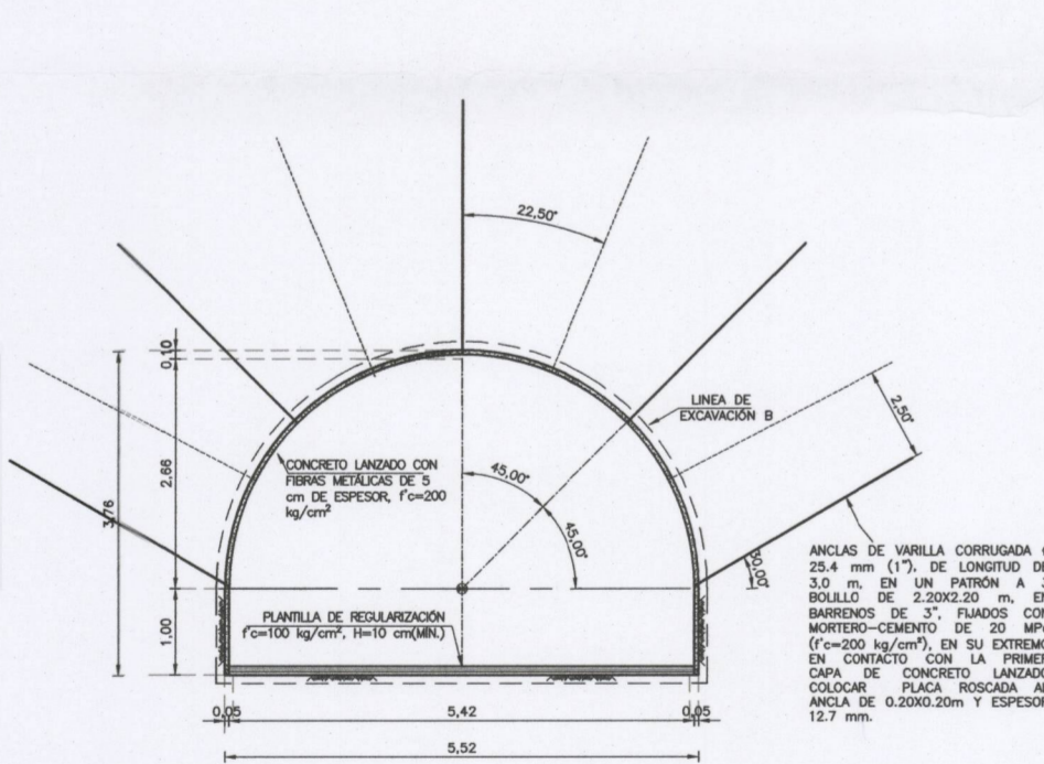
GALERÍA DE APROXIMACIÓN-TIPO A ESC. 1:100
