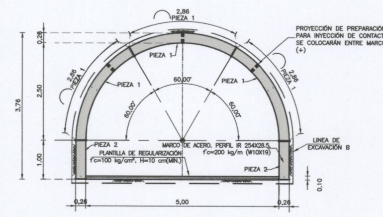
GALERÍA DE APROXIMACIÓN-TIPO C ESC. 1:100
